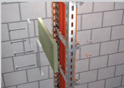
Montáž opěrné desky pomocí šroubů se šestihlannou hlavou na zavěšenou stoupací trasu.
