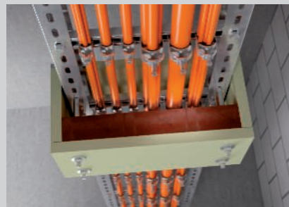
Zaplnění namontovaného pouzdra pěnovými bloky PYROPLUG® Block.
