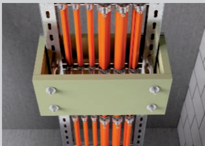
Kompletně namontované pouzdro.
