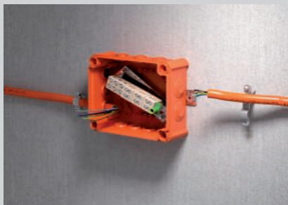
Zavedení kabelů přes násuvná těsnění.
