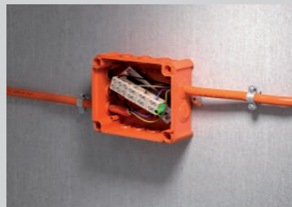
Úhlopříčně umístěná svorkovnice s velkým zapojovacím prostorem.
